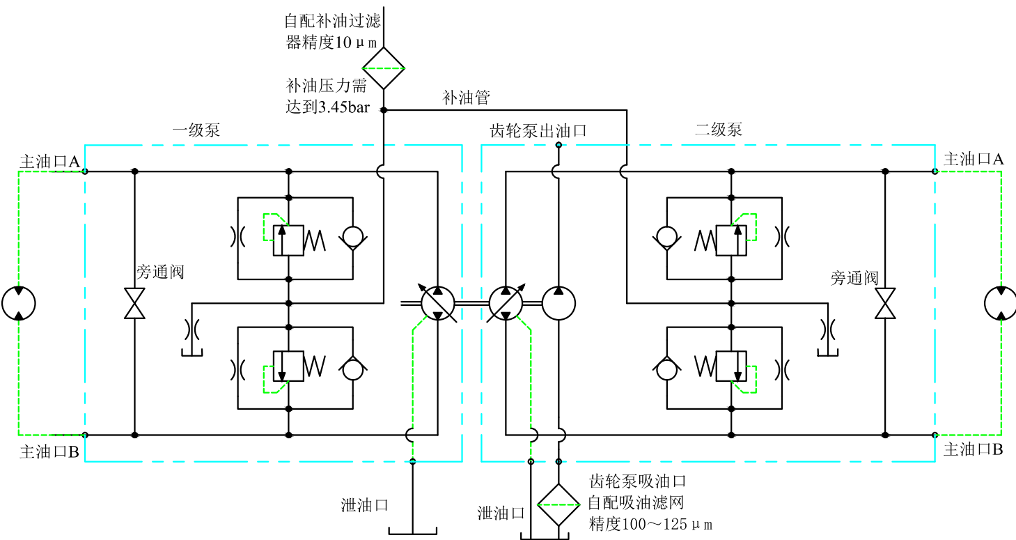
双泵连齿轮泵回路图
