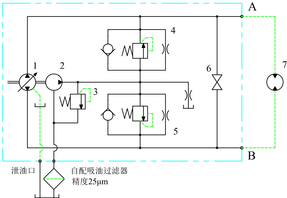
单泵连齿轮泵回路图
