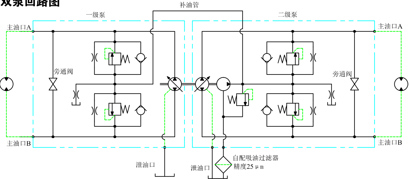
双泵连齿轮泵回路图
